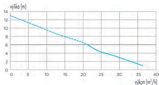
Oběžné kolo Vortex KX V6
