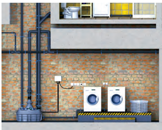
Externí vzdálený alarm
