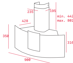
DU 985 EP CRISTAL
